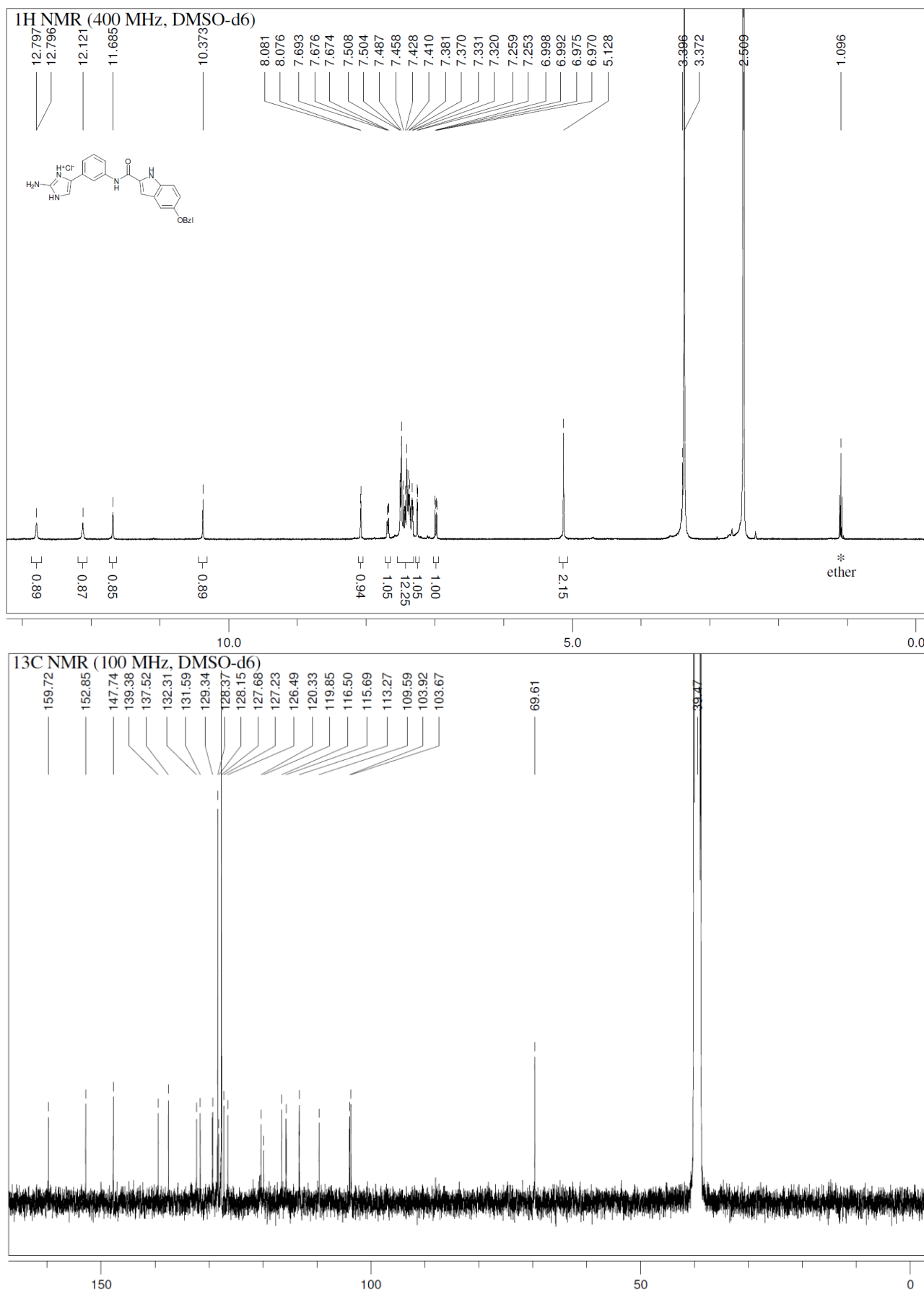
Figure S13. 2-Amino-4-(3-(5-(benzyloxy)-1H-indole-2-carboxamido)phenyl)-1H-imidazol-3-ium chloride ( 6h ).
