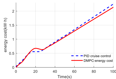
(d) Comparison result of energy consumption
