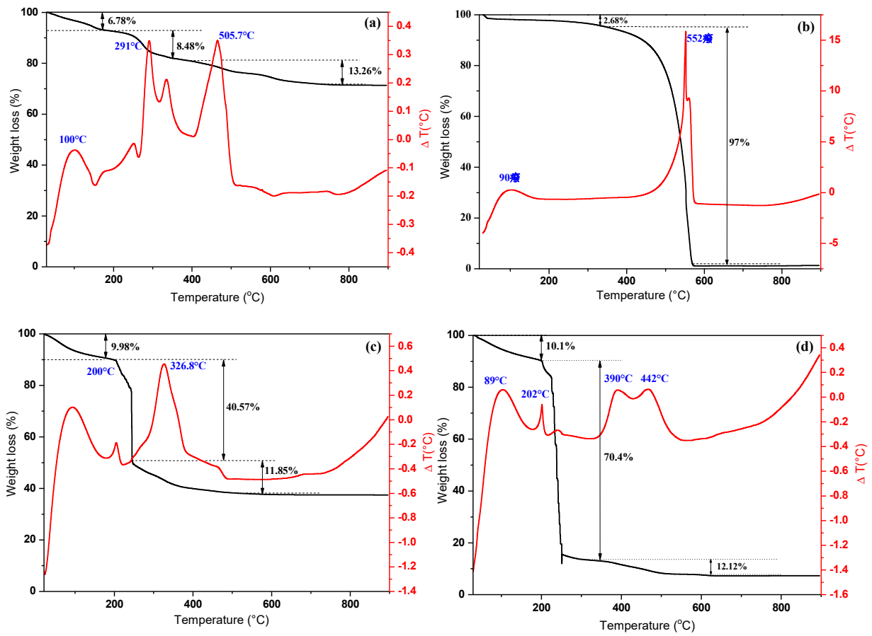
Figure S1. TGA/DTG profiles of (a) \gamma -Fe 2 O 3 particles, (b) f-CNT, (c) A/ \gamma -Fe 2 O 3 , (d) A/ \gamma -Fe 2 O 3 /f-CNT beads.
