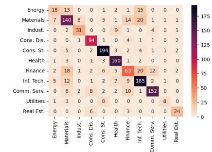
(d) One-vs-Rest with autoencoder for dimensionality reduction
