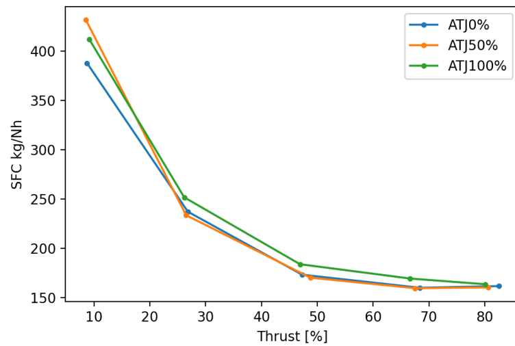
Figure 12. GTM-140/ATJ: SFC.
