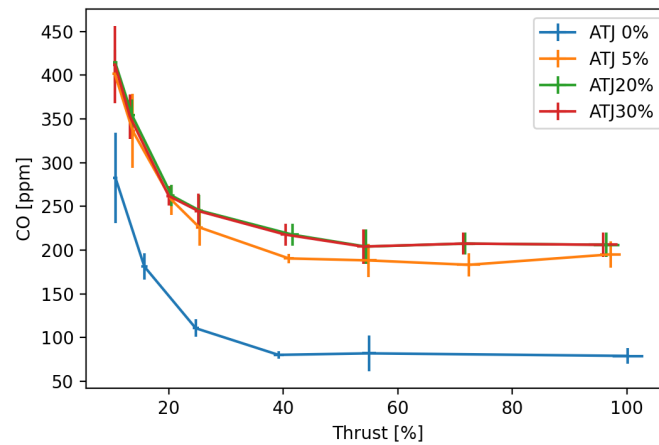
Figure 29. DGEN 380/ATJ: CO.
