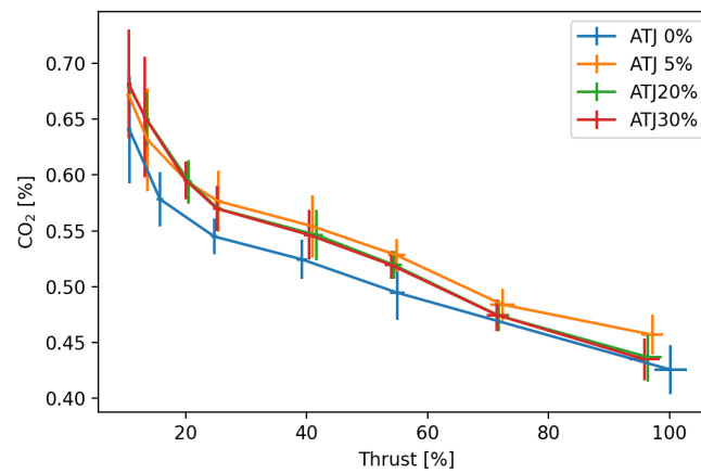
Figure 30. DGEN 380/ATJ: CO 2 .
