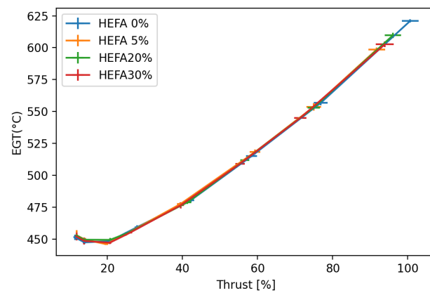
Figure 28. DGEN 380/HEFA: EGT.
