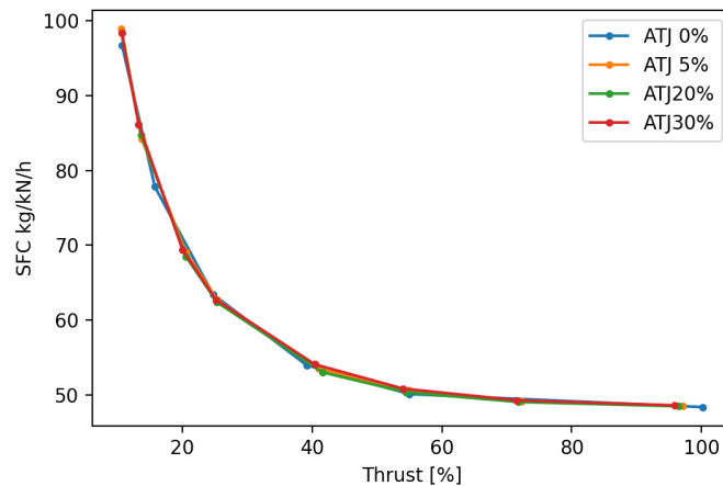
Figure 25. DGEN 380/ATJ: SFC.
