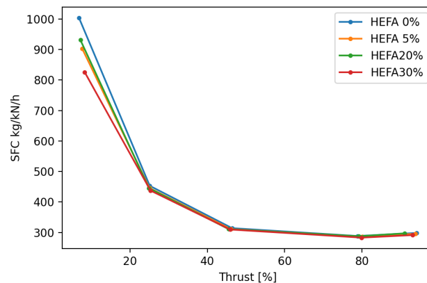
Figure 18. GTM-140/HEFA: SFC.
