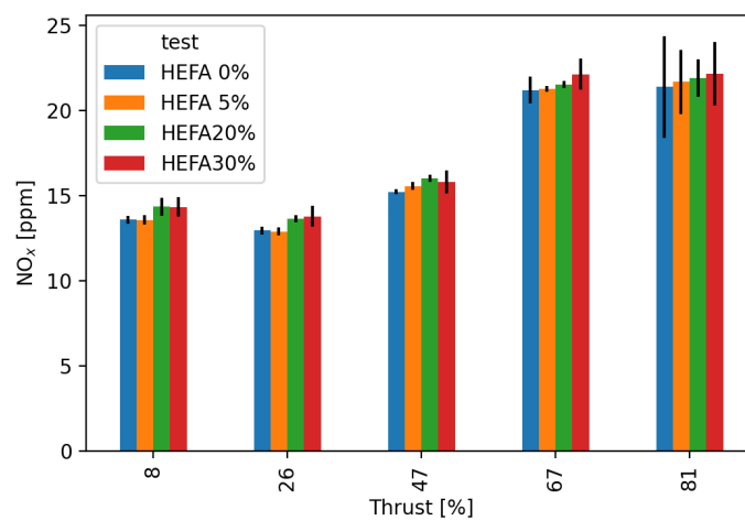
Figure 21. GTM-140/HEFA: NO x .
