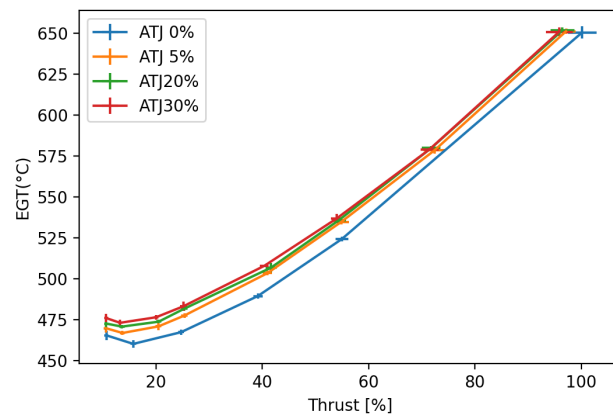
Figure 27. DGEN 380/ATJ: EGT.
